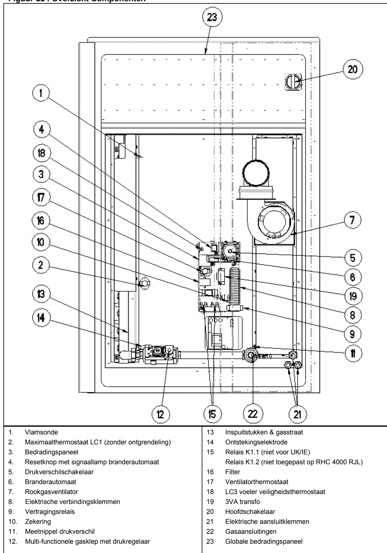
Figuur 11 : Overzicht Componenten
