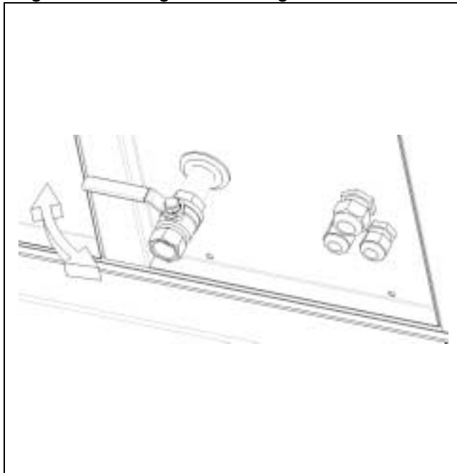
Figuur 3 : Detail gasaansluiting
