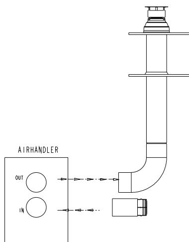
Figuur 2 : Systemen voor toevoer verbrandingslucht & afvoer verbrandingsgassen
