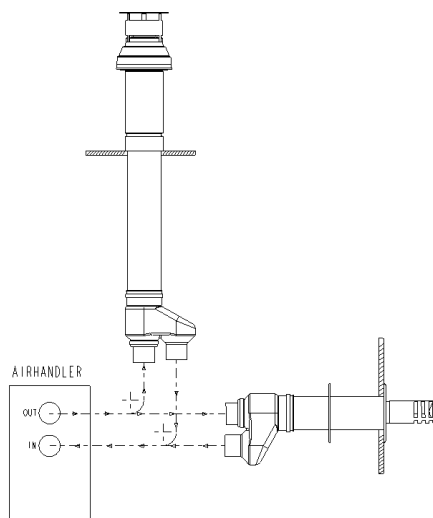
Figuur 1 : Systemen voor toevoer verbrandingslucht & afvoer verbrandingsgassen
