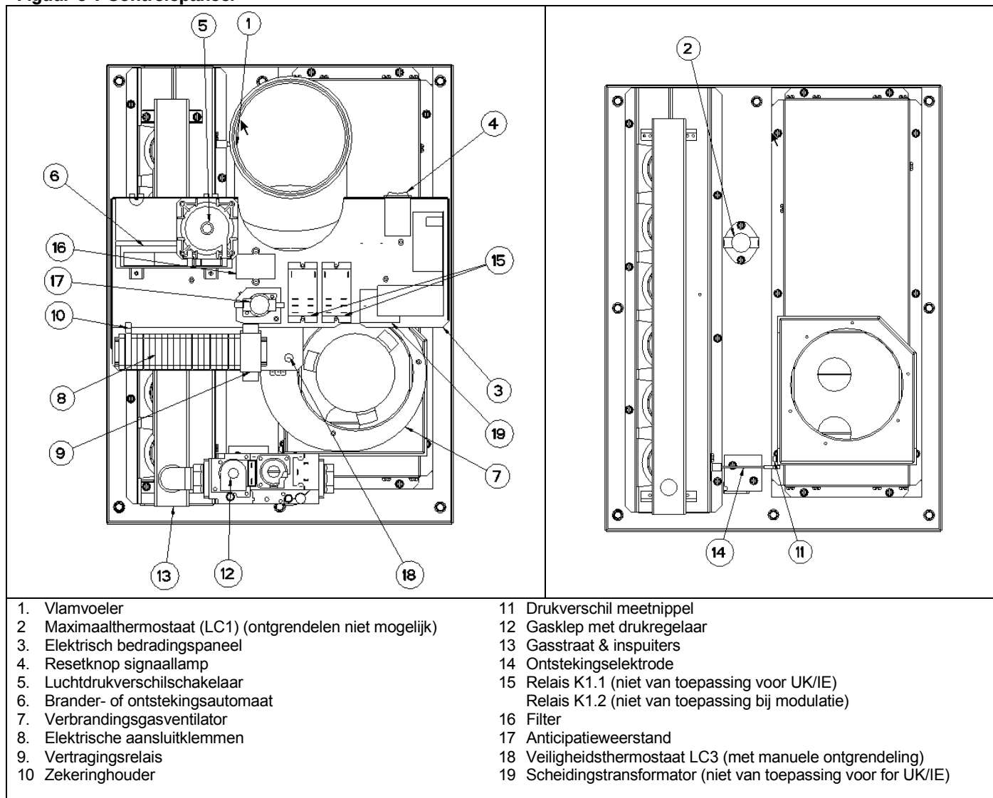
Figuur 9 : Controlepaneel
